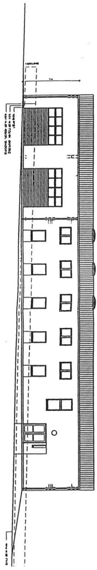
OSTANSICHT
